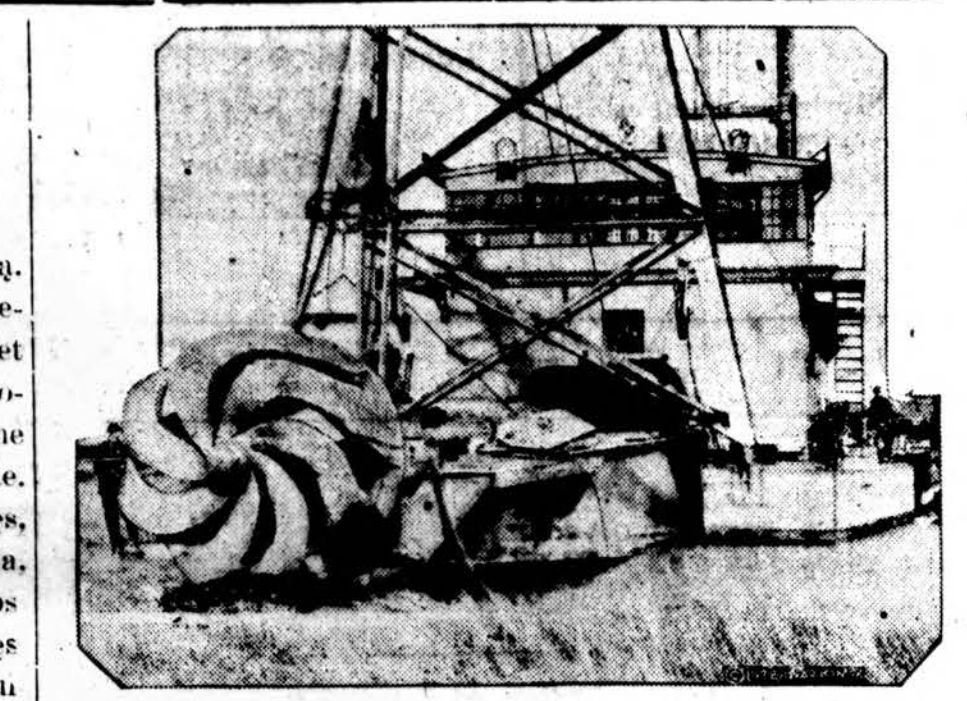
Milžiniška mašina upės dugnui gilinti. Ši mašina paleista darban ant St. Lawrence upės tarpe St. Louis ir St. Francis ežerų. Mašina kasdien iškasa po 200 pėdų žemės. Neužilgo bus iškastas kanalas 300 pėdų pločio ir 27 pėdas gilumo. Kanalas bus dalis St. Lawrence vandens kelio.
