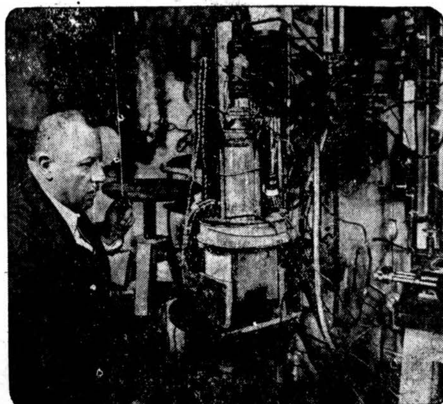
Leyden'o universiteto, Olandijoje, prof. dr. W. H. Keesom pranešė, kad jam pavyko dešimtis kubinių centimetrų tuštumą atšaldyti ligi 0.75 K laipsnių, kas yra lygu — 489 laipsniais Fahrenheito termometro. Tas yra arti absoliučio šaltio zero. Tos rūšies žema temperatūra dar nebuvo atsiektą.
