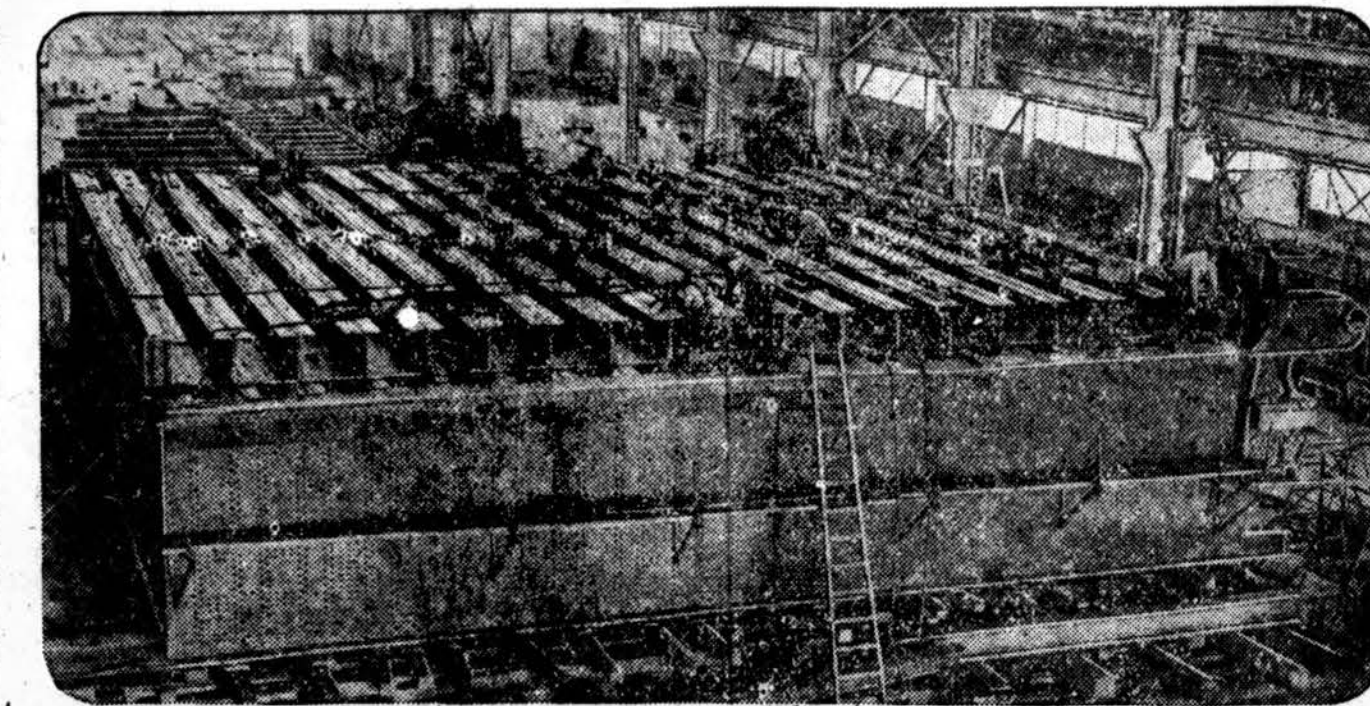
Hoover'io užtvankos Colorado upėje vieni milžiniški plieno vartai jau padirbdinti. Užtvanka dirbama laukų drėkinimo reikalam.
