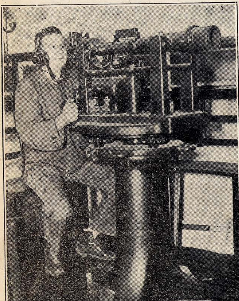
Čia matome instrumentą, kuriuo susekamas priešininko laivas jūroje. Toks instrumentas randasi Fort Hamilton, Brooklyne. Šitaip susekus priešininko laivo pozicija galima prisitaikyti jį bombarduoti.
