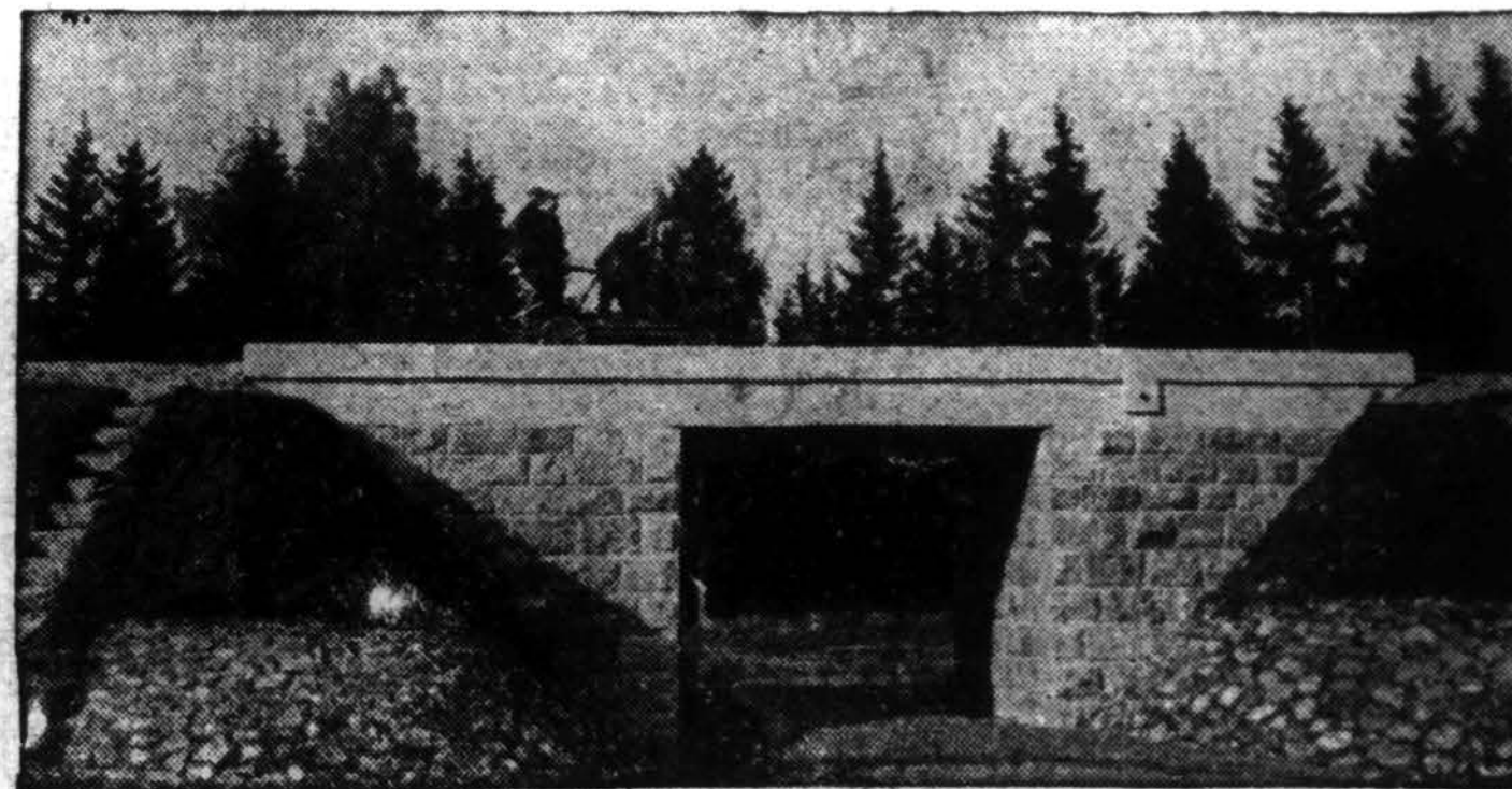
Lietuvos pažangos liūdytojas. Surviliškio tiltas per Nevėžį (Kėdainių apskrity). Tiltas yra savotiškos konstrukcijos ir gražios gamtos aplinkumoje sudaro puikų vaizdą.
