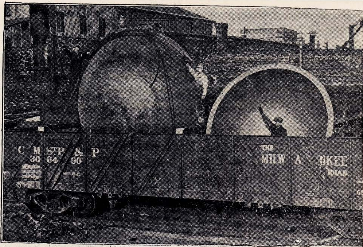
Tai bent katilai. Chicagoj nuliedinti ir į Kellogg, Idaho išsiųsti šie milžiniški švinui virinti katilai. Kairėj katilas turi 16 ir pusę pėdų diametre ir sveria 20 tonų. Jame galima bus vienu sykiu suvirinti 235 tonos švino.
