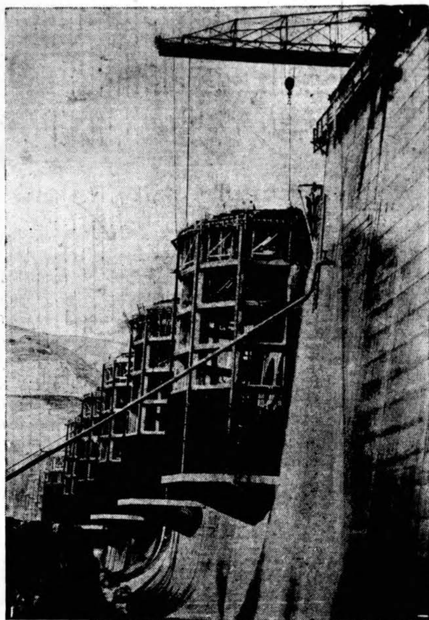
Grand Coulee gelžbetoninė užtvanka Columbia upėje.
