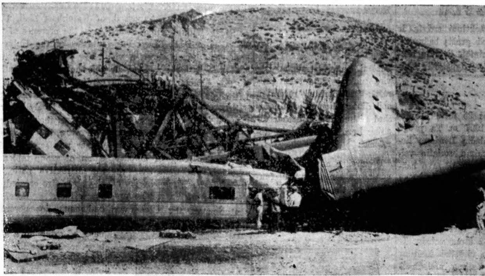
Liukusinio traukinio "City of San Francisco" penki kelei viniai vagonai per katastrofą suvirtę viens ant kito lyg krūva dėžių. Užpakaly sulaužytas ir geležinis tiltas per upę. Kiti vagonai nušokę nuo bėgių sudužo ir nuo status kran- to nusirito į upę. (Acme telephoto)
