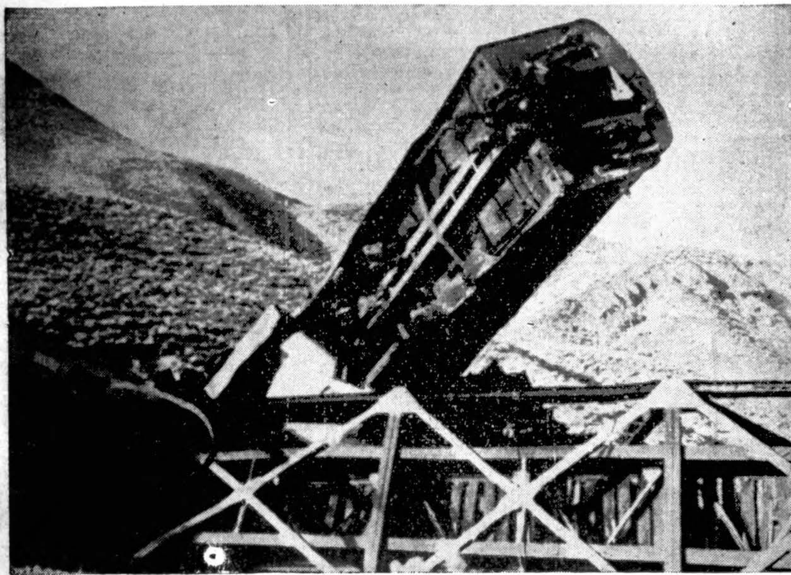
City of San Francisco traukinio nelaimėje Nevados dykumose 23 asmenys žuvo ir daugiau kaip 100 kitų keleivių sužeista. Southern Pacific geležinkelio kompanijos viršininkai ir koronerio teismo prisėdai tvirtina, kad nelaimė įvyko dėl sugadintų bėgių. Koks pakvaišėlis galėjo tai atlikti. Vienas įtariamas suimtas. (Aeme telephoto).
