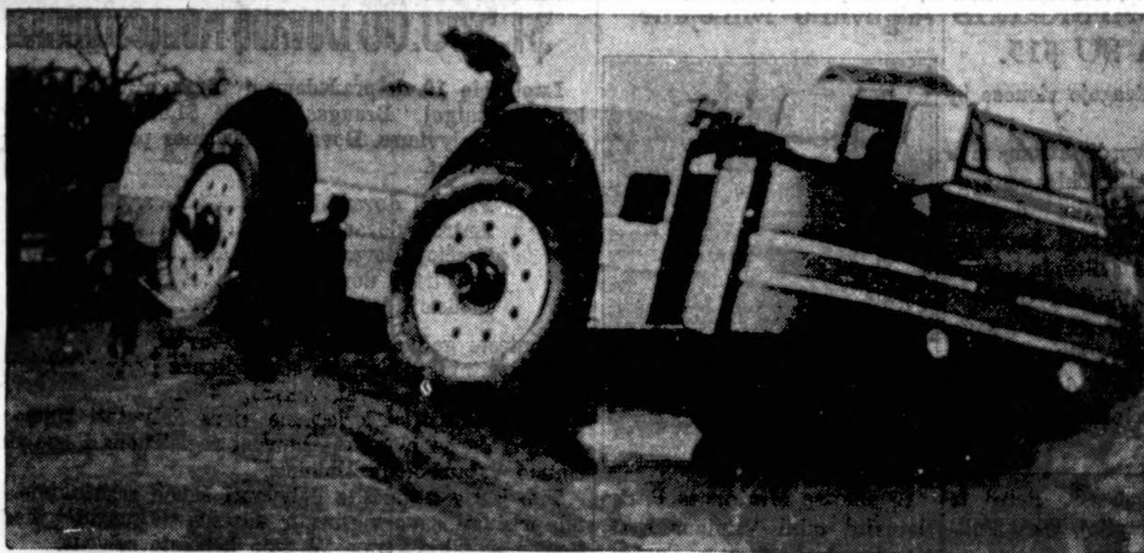
„Sniego kreiseris“ (milžiniškas sunkvežimis), Armouro Instituto Fondacijos Chicagoje, lėšomis padirbdintas admiralu Byrd ekspedicijai į pietinį žemės ašigalį. Po sėkmingo išbandymo Indiana smėlynuose, sunkvežimis važiuavo į Bostoną, kur jo laukia paruoštas ekspedicijai laivas. Netoli Lima, Ohio, važiuojant per upelį, tiltas milžino neatlaikė, lūžo ir „sniego kreiserį“ matom įvirtusį į griovį. (Acme telephoto)
