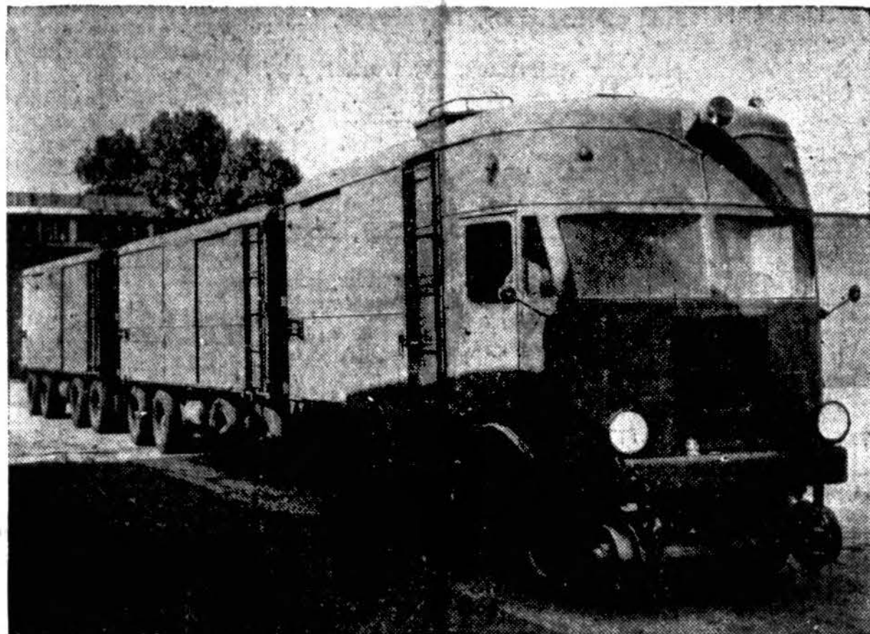
Highland, Ill., padirbdintas auto-vagonas, kuriuo galima važiuoti paprastuoju planu, o, prireikus, ir geležinkelio bėgiais. Siunčiamas į ordinanso dirbtuvę.
