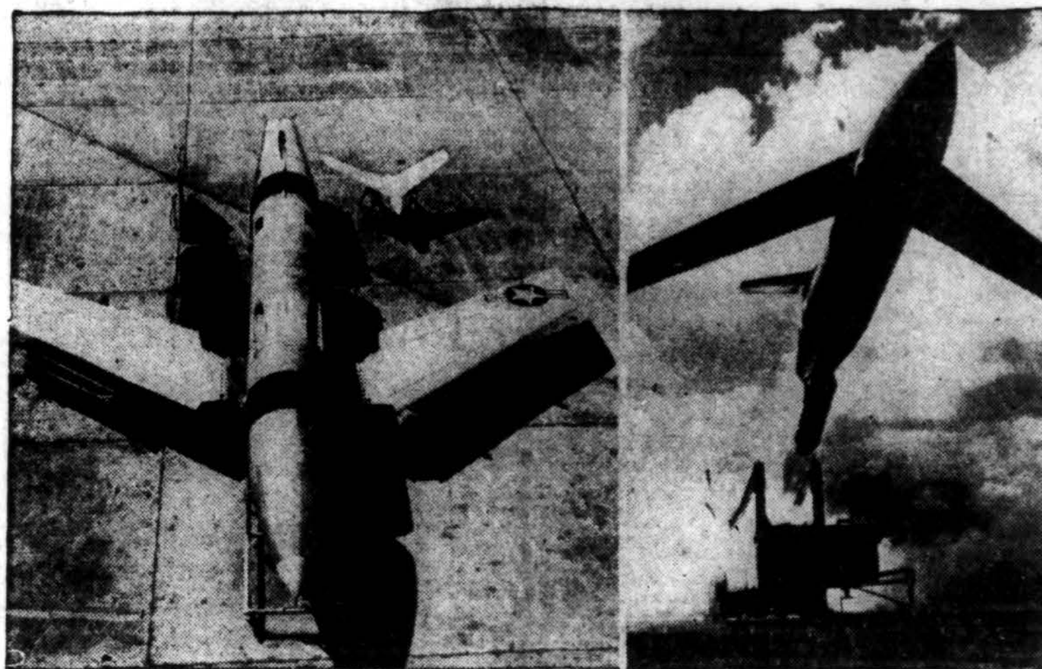
Bepilotinis bombonešis B-61 Matador yra taip padarytas, kad gali būti pervežtas atskiromis dalimis ir sumontuotas ten, iš kur turi būti paleistas skristi į taikinį. Kairėje matomas bombonešio sumontavimas, o dešinėje — pakilimas nuo mažiausio pasaulio aerodromo, kuriuo yra jo iššovimo platforma. (INS)
