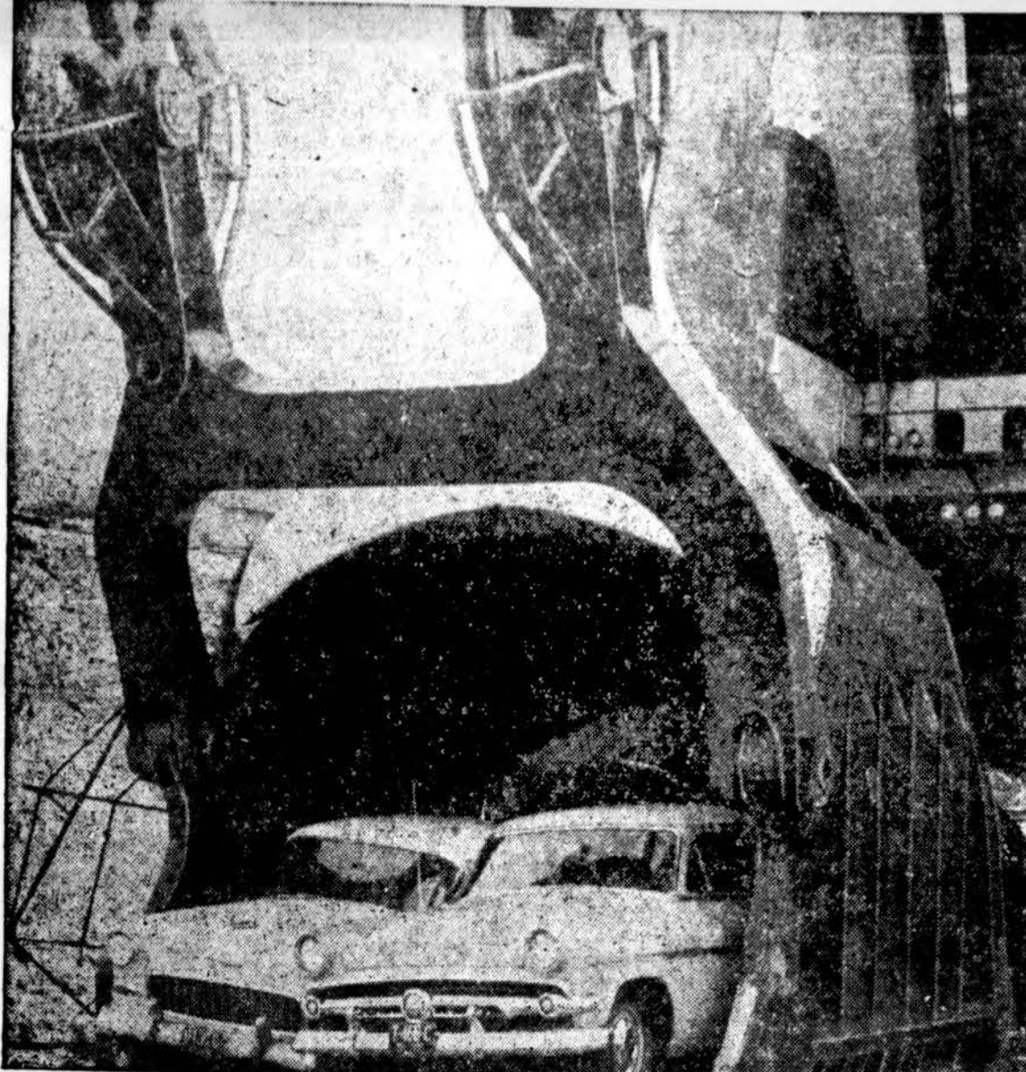
— Du automobiliai pastatyti vienas šalia kito didžiulėje kasimo šiupeleje, kuri vienu pašimtu iškasa 16 tonų anglies. Tos mašinos atskiras dalis iš Marion dirbtuvės, Ohio, vežė 125 vagonai į Hanna Coal kompanijos Georgetown anglies kasyklas, netoli Cadiz, Ohio.
