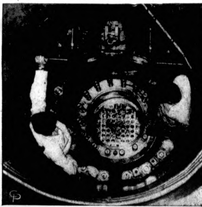
Taip iš viršaus atrodo atdaras kariuomenės sudarytas atominis reaktorius, esąs Belvoire, Va. Jį galima paversti sunkvežimiu ar perkelti lėktuvu. Vidury matomos duobutės yra vieta atomiškai besiskaidančioms medžiagoms. Šis reaktorius gamina elektrą.
