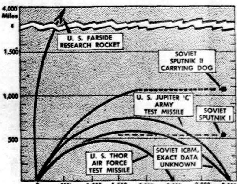
Raketų tolis. Brėžinys palygina sovietų raketų pasiekimų augimą ir tolimą su Jungtinių Amerikos Valstybių išbandytomis ir būsimomis raketomis. „Operation Far Side“ raketa, neseniai išbandyta JAV, išsauta 4,000 mylių į erdvę. Sovietų Sputnik II yra tik 1,000 mylių erdvėje. (INS)
