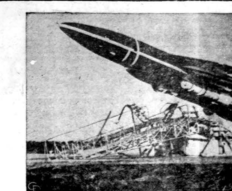
JAV aviacijos tarptautinė „Snark“ strateginė raketa. Ji pakyla nuo raketos platformos. Po raketos sparnais yra pagalbiniai skystojo kuro raketiniai jėgos keliaviečiai, pristatant atominę galutinę. (INS)
