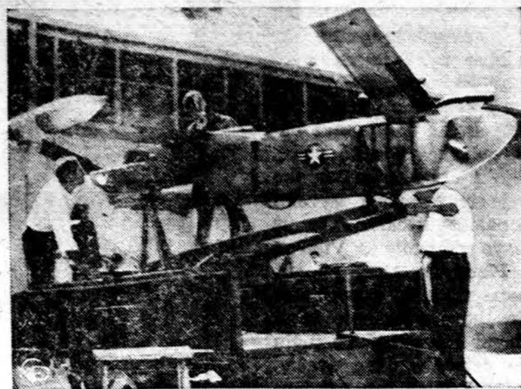
Vaižde matyti naujas bepilotinis lėktuvas prieš pozicijoms tirti. Lėktuvas paleidžiamas nuo sunkvežimio platformos dviejų raketų pagalba, kontroliuojamas nuo žemės ir jon grįžta parašiuo pabalba.
