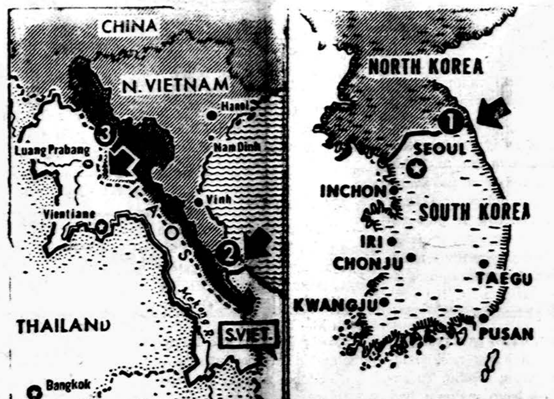
Laose galimais daiktas bus pasiekta tas, kas yra daugelyje kitų valstybių — ji bus padalinta. 1953 m. buvo padalinta į dvi dalis Korėja (1), 1954 m. Viet Nam (2) ir dabar Laos (3). Be dviejų Kinijų, dviejų Vokietijų, dviejų Korėjų galimais daiktas turėsime ir du Laosus. (UPI)
