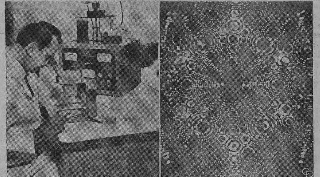
Atomai, padidinti 2,700,000 kartų. Naujas ypatingo galingumo Muller Field ionų mikroskopas parodo dabar atskirus atomus, kurių anksčiau nebuvo galima matyti. Kairėje matome Chicagos mokslininką, kuris naudojamas paprastu mikroskopu atskiria dalelytę metalo, paskiau dešinėje parodoma per naująjį mikroskopą. Matomas beveik tobulas tungsteno kristalas; taškai, kurie sudaro tą "piešinį", yra atomai, padidinti 2,700,000 kartų.
