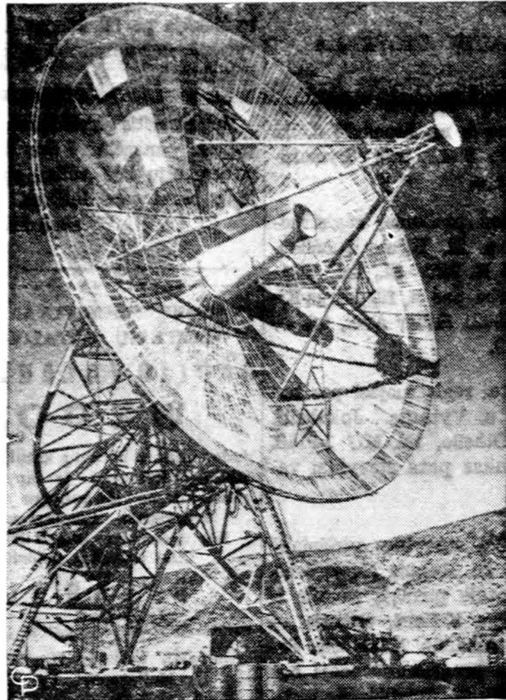
Didžiulė 85 pėdų antena įrengta Deep Space Tracking stotyje Californijoje, kuri priims nuotraukas, siunčias Mariner 4 raketos iš Marso. Vienos nuotraukos atėjimas iš Marso užtrunka net aštuonias valandas 35 minutes, nes tai yra 134 mil. mylių nuotolis.
