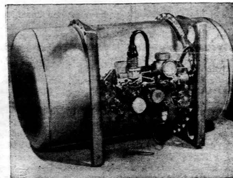
Elektros celė. Šioje nuotraukoje parodyta elektros celė, kuri bus naudojama valdant Gemini-5 kapsulę. Elektros celė pakeičia baterijas. Dabar vietoje baterijų yra šios rūšies du aparatai.
