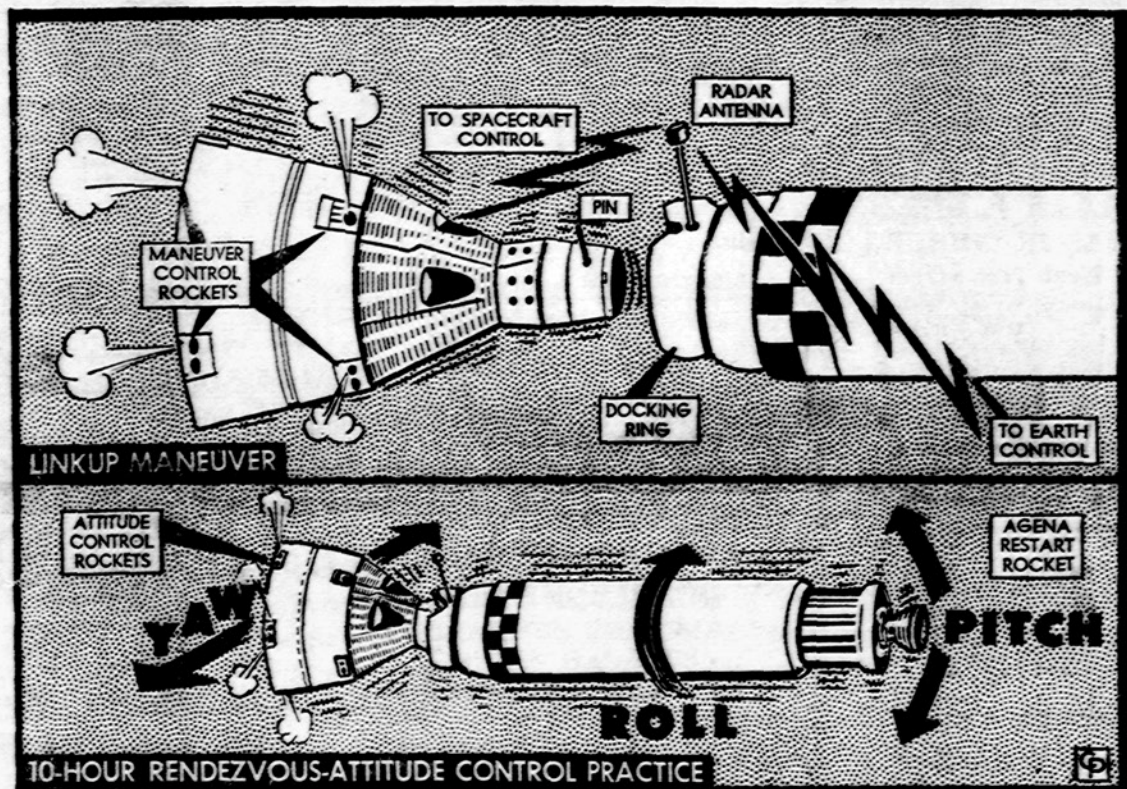
Susijungimo manevrai. Brėžiniai rodo kokiais manevrais erdvės laivas Gemini-6 kels kartus susijungus su raketa Agena. Viršuje rodoma kaip laivo nosis turės įlysti į Jungtinio ratą. Apačioje rodoma kaip susijungtas vienetas bus manevruojamas aštuoniomis erdvės laivo mažesniais raketomis.
