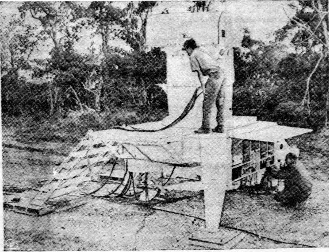
Nuotraukoje parodytas vadinamas laser persiuntimo ir priėmimo aparatas sekimo ir priėmimo stotyje Kokee, Kanai, Havajų salose, kur buvo užmegztas ryšys su kosminiu laivu Gemini-7. Fred H. Shigemoto yra ant platformos ir Kent R. Bourquin prie instrumentų pulto. Abu yra mokslininkai.
