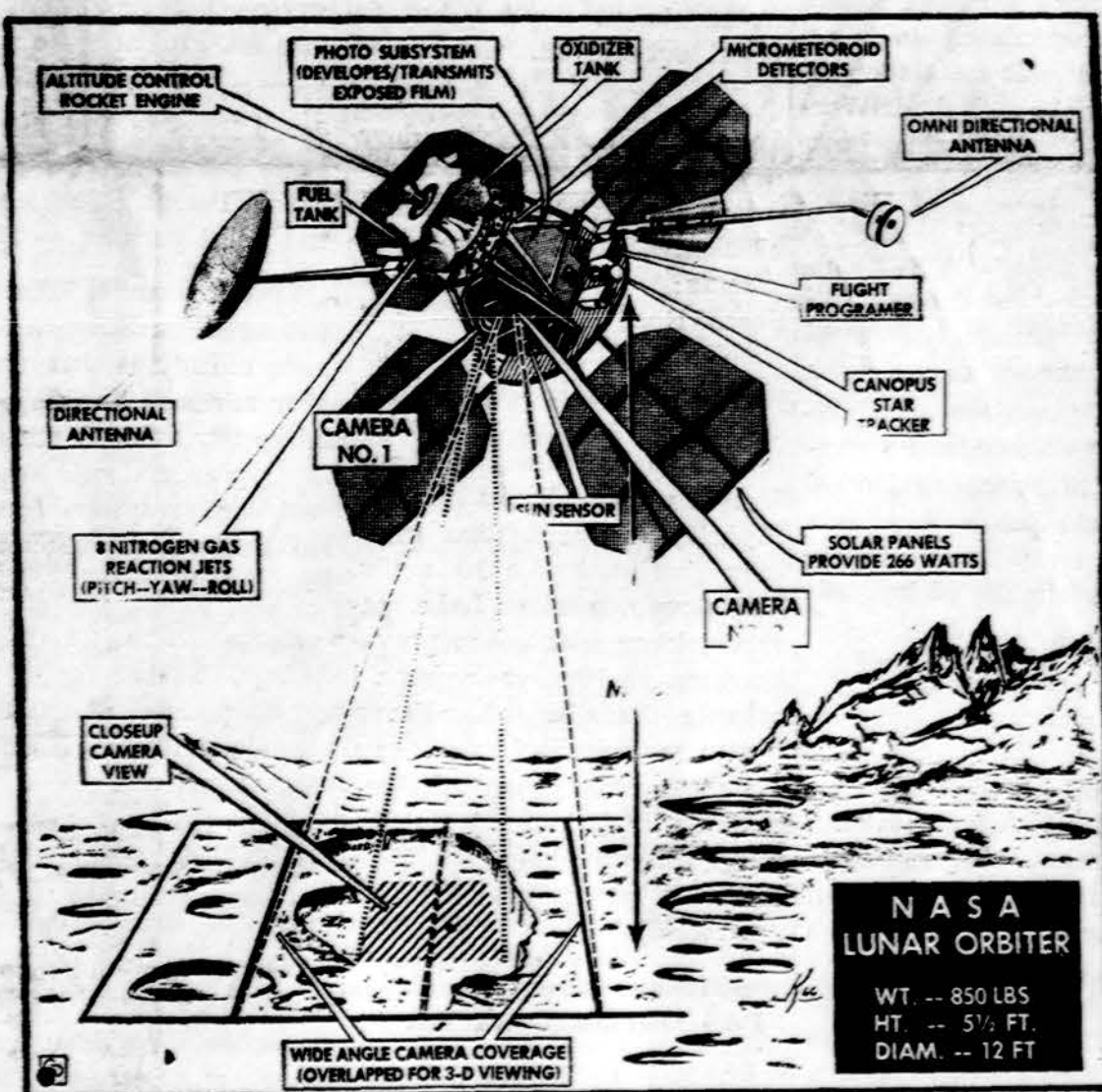
Šis brėžinys pavaizduoja JAV-ų „Lunar Orbiter“ mechanizmą ir jo darbą. Erdvėlaivis „Lunar Orbiter“ skrieja aplink Mėnulį ir daro jo paviršiaus nuotraukas. Šis erdvėlaivis padarys nuotraukų tų vietų, kuriose numatomas JAV-ų astronautų nusileidimas.
