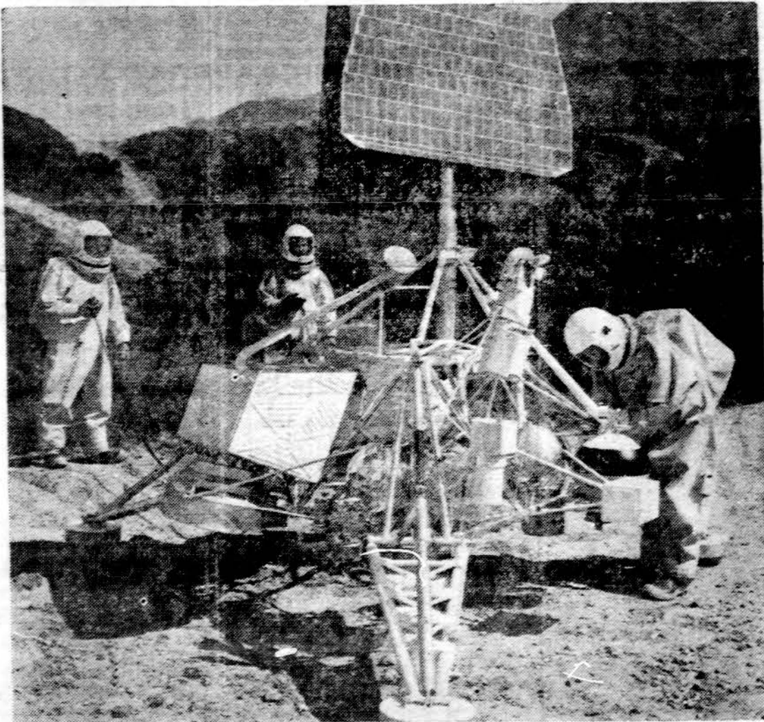
Erdvėlaivio Surveyorio II išbandymas. — San Gabriel kalnuose Kalifornijoje Hughes aviacijos technikai bando Surveyorio II modelį, patikrindami motoro sistemą, kuri turės nuleisti šį erdvėlaivį minštai ant Mėnulio paviršiaus. Erdvėlaivis I, esąs ant Mėnulio nuo praėjusio pavasario, atsiumė Žemėn daugiau kaip 11,000 Mėnulio paviršiaus noutraukų. Surveyor II numatytas rugsėjo 20 d. iš Cape Kennedy bazės paleisti ant Mėnulio.
