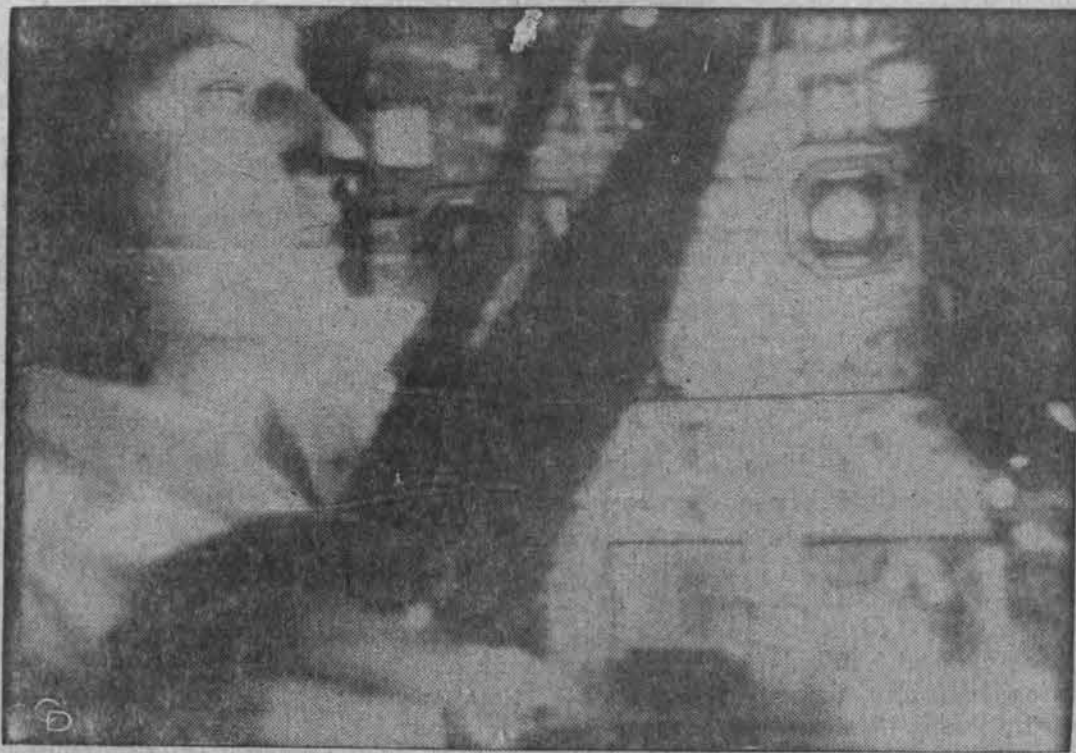
Iš erdvėlaivio Apollo 12 perduodamas vaizdas per televiziją. Vaizde astronautas Charles Conrad.
