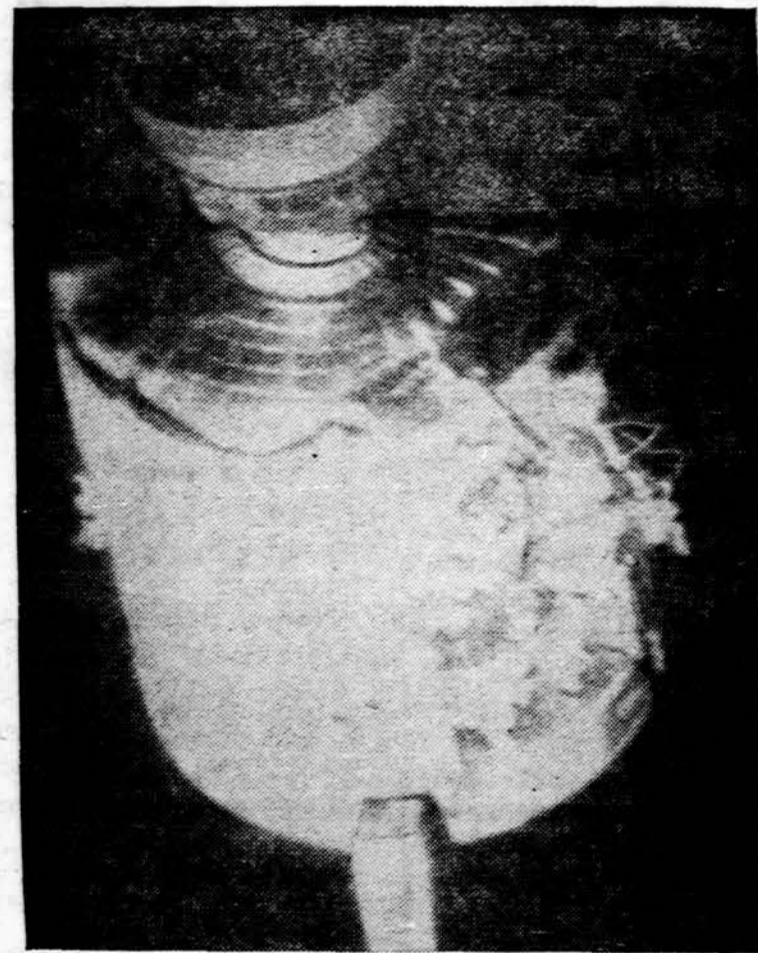
Apollo 13 astronautai padarė šią erdvėlaivio priekabos nuotrauką kai ją atskyrė ir ji ėmė tolti. Dešinėje matyti susprogęs šonas.
