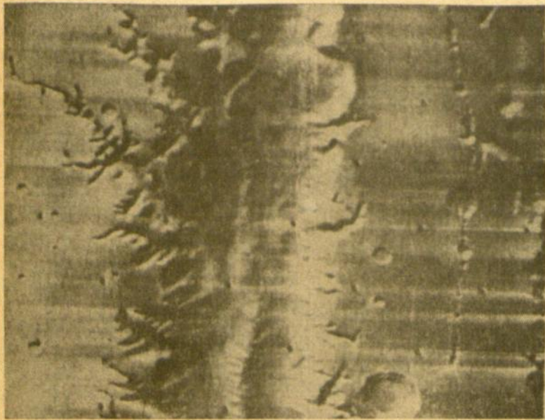
Coprates slėnio dalis, fotografuota Mariner 9-tojo iš 1225 mylių aukščio
