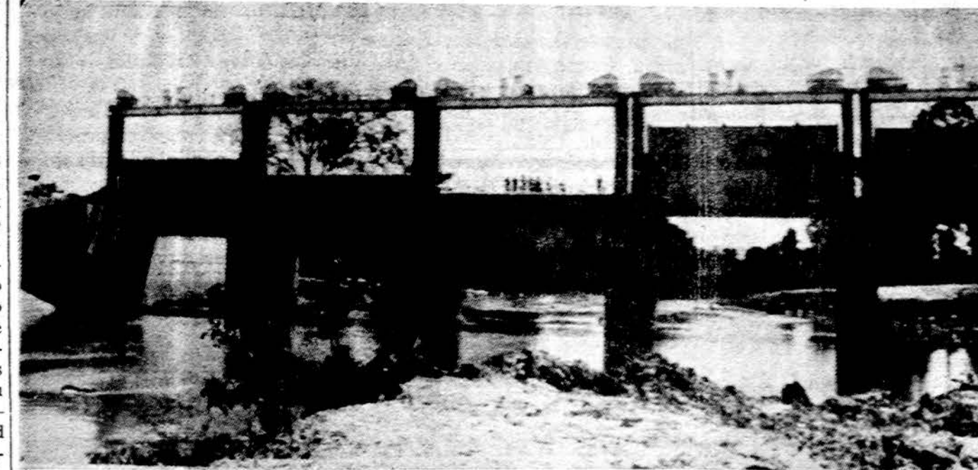
Amerika, kariaudama Indokinijoje, ne tik grynė kraštą nuo komunizmo, bet tiesė kelius, statė įvairius pastatus. Čia matome JAV ir Japonijos lėšomis pastatytus užtvankos įrengimus prie Prek Thnot, Kambodijoje.
