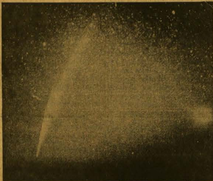
Šeštoji 1970 metų kometa, 1970f, Zodiako šviesoje. Šią kometa nepriklausomai surado trys asmenys, tad ir kometa vadinama White-Ortiz-Bolelli. Graeme L. White tuo metu buvo 22 metų amžiaus universiteto studentas Australijoje, Emilio Ortiz prancūzų lėktuvų kompanijos antrasis pilotas, pastebėjęs kometa, skridamas 70 raketiniu lėktuvu viršum Indijos vandenyno, o Carlos Bolelli, astronomas, surado ją Čilėje.
