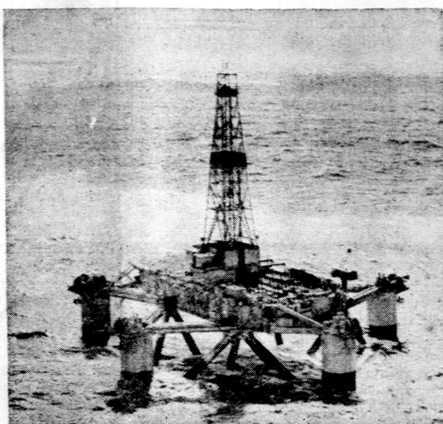
Shell/Esso įrengta naftos pumpavimo stotis šiaurės jūroje
