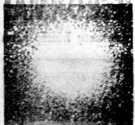
Rutininis uždaras žvaigždžių spiečius M13 Herkulo žvaigždynė. Iki 1974 metais pasijuti radio signalai. Spiečius priklauso Paukščių Tako galaktikai.
