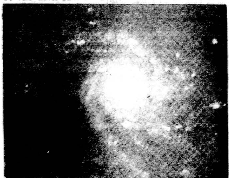
Ispūdinga spiralinė galaktika Berenikės Kasų žvaigždynė
