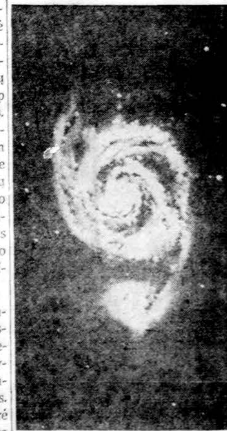
Astronomams gerai pažįstama galaktika M 51 Skalių žvaigždynė. Jau 1860 metais Lordas Rosse įžūrėjo jos spiralinę struktūrą. Maždaug tokio pat dydžio, kaip ir Paukščių Takas. Apacių matyt gana masyvi patalvė nereguliarios struktūros galaktika, susijungusi su pagrindine lyg ir žvaigždžių tūlu. Ši įdomi galaktika vadinama Verpetu (Whirlpool).
