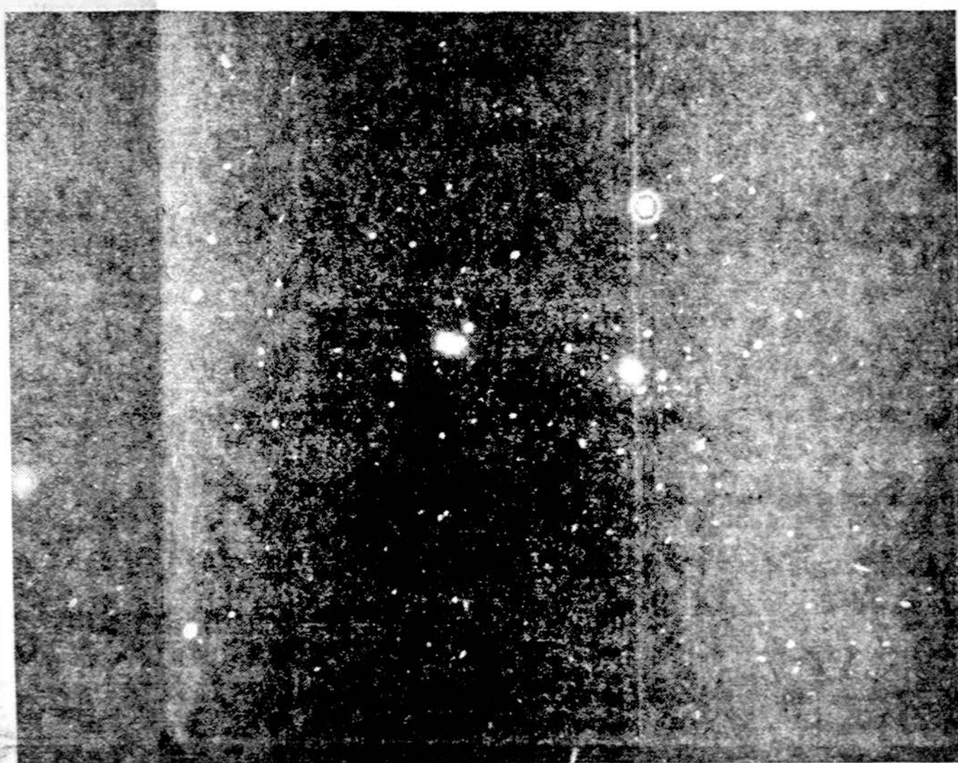
Čia ne žvaigždės, o didžiulis spiečius galaktikų Berenikės Kasų žvaigždynė. Kiekviena švieselė tai vis atskiras Paukščių Takas, atskira galaktika. Tikima, kad iki jų yra 300 milijonų šviesmečių. Argi ne vienoje iš tų galaktikų nėra gyvybės?
