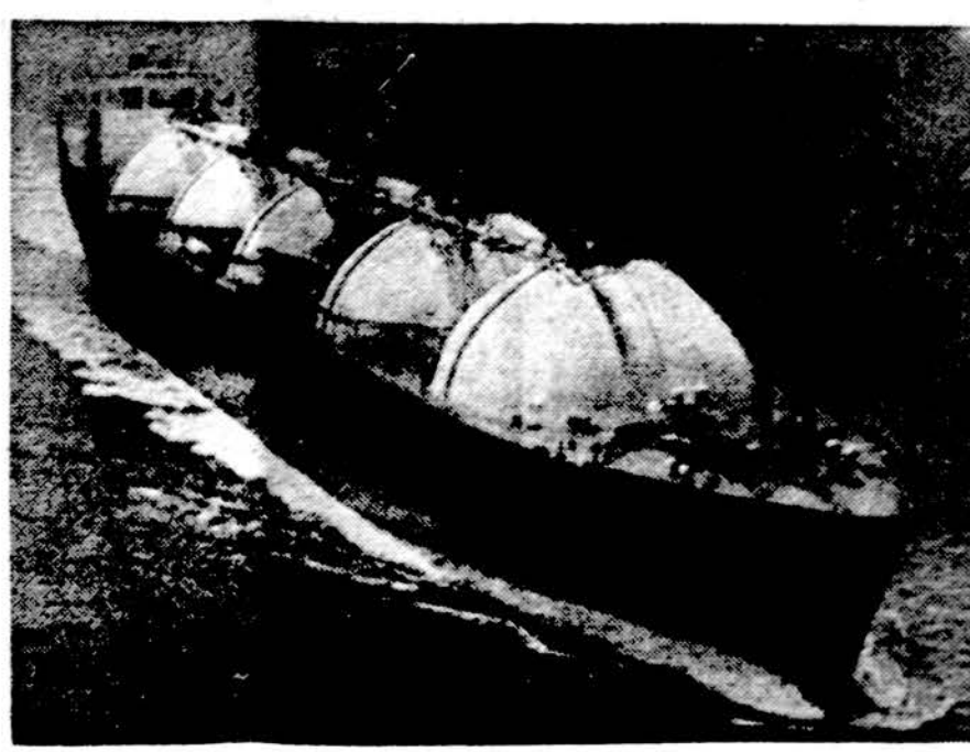
Suskytintoms dujoms gabenti tankas
