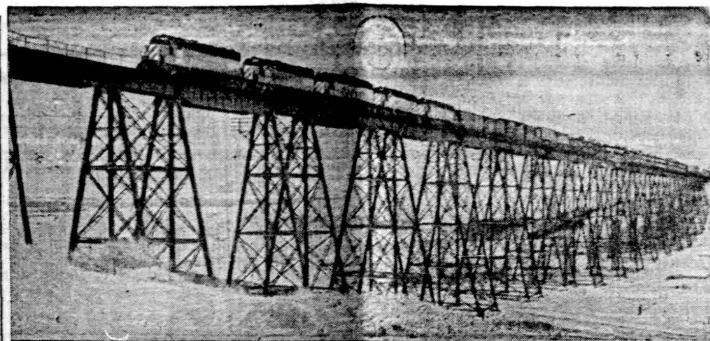
Burlington Northern geležinkelio Co. traukinyje, traukiamas penkių garvežių, rieda Gasman Coulee tiltu, North Dakota. Šis tiltas ištiestas per silėnį yra 1,792 pėdų ilgio ir 117 pėdų aukštumo
