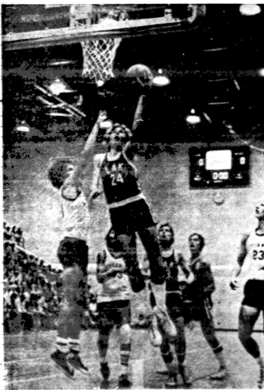
R. Šimkus "sodina."
