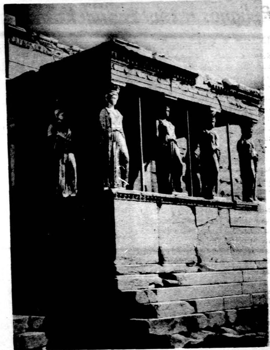
Klasikinė Graikija — Erechtojo šventyklos korintiškos stulpai
