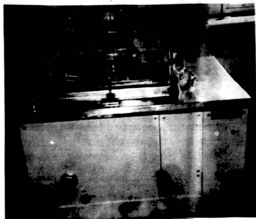
ALIDCORP filialas Šeduvoje plečia žemės ūkio veiklą į sūrio, sviesto ir grietinės gamybą. Nuotraukoje - sūriui gaminimo įranga - nerūdijantis pieno, garų šildomas 240 litrų katilas.
