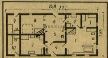
Iš Igno Jablonskio „Budrių kaimas“, 6 pavyzdys. Jono Šikšniaus trobos, statytos 18-ojo amžiaus pirmoje pusėje, planas: 1 — geroji troba, 2 — užpeinė, 3 — alkierius, 4 — geroji priemenė, 5 — kaminas, 6 — prastoji priemenė, 7 — priešininkė, 8 — dūminė, 9, 10 — kambaras.
