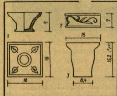
Iš Igno Jablonskio „Budrių kaimas“, 28 pavyzdys. 1 — krosnies kolkis (puodinė) Jablonskio senojoje troboje (18 a.), 2 — krosnies detalė Jablonskio troboje (18 a.), 3 — kolkio (puodinės) schema iš Daukšinio senosios trobos (17 a.)
