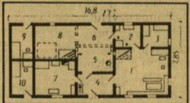
Iš Igno Jablonskio „Budrių kaimas“, 6 pavyzdys. Jono Šikšniaus trobos, statytos 18-ojo amžiaus pirmoje pusėje, planas: 1 — geroji troba, 2 — užpeinė, 3 — alkierius, 4 — geroji priemenė, 5 — kambaras, 6 — prastoji priemenė, 7 — priešininkė, 8 — dūminė, 9, 10 — kambaras.
