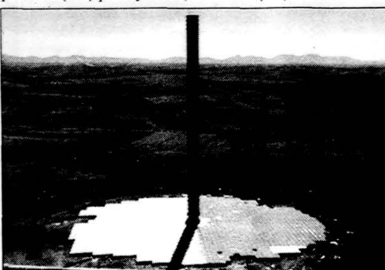
Saulės bokšto prototipas (50 kW) veike Ispanijoje 1982–1989 m.
