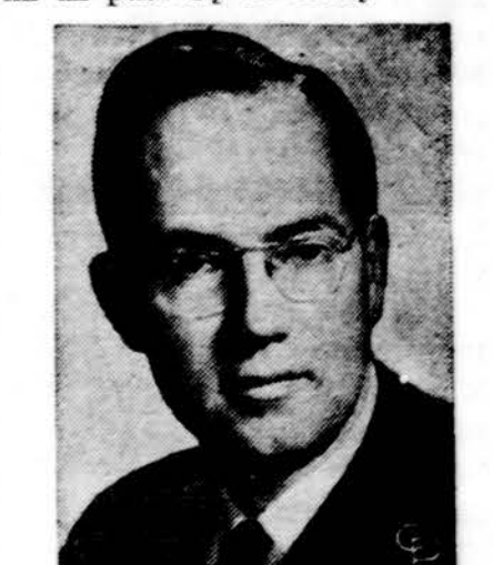
Dr. Charles H. Townes, Massachu- setts Technologijos instituto pro- fesorius, paskirtas Nobelio premija fizikos srityje. Jis tapo premija ($53,123) pasidalins su dviem Maskvos universiteto profesorais. Townes premija paskirta dėl kie- kio elektronikos pagrindų tyrinė- jimo, kurio dėka buvo padirbtos, Maser-Laser principu pagrįstos, šviesos spinduliuotės stiprinimo. Maser vadinasi "mikrobanginis spinduli- vimo stiprinimas paskaita sklai- da". (UPI)
