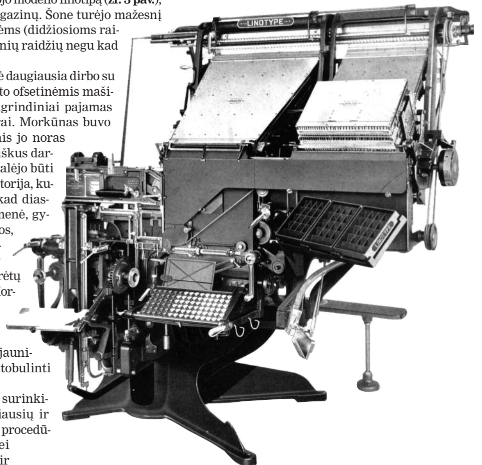
3 pav. Keturioliktasis linotipo modelis, kokį iš pradžių turėjo Mykolo Morkūno spaustuvė (Fot. http://linotyperegistry.org/models/mlc/14/prev_model14.png )
