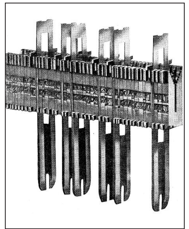
2 pav. Surinkta matricų eilutė su tarpais tarp žodžių (Linotype Machine Principles 1940, 8)
