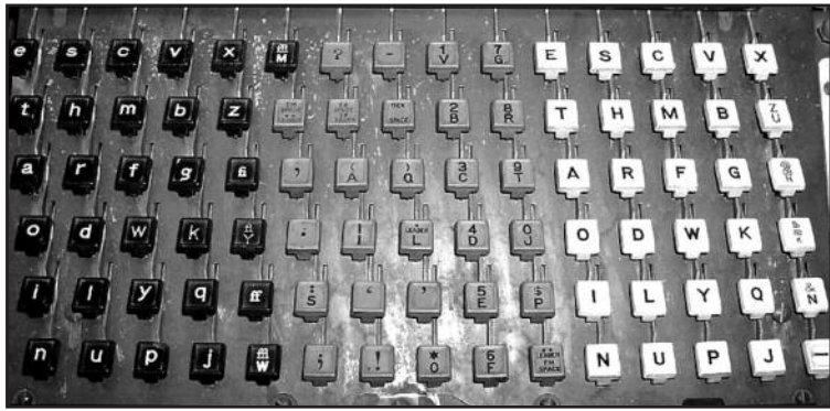
4 pav. Linotipo mašinos klaviatūra. Pačioje kairėje (juodi klavišai, baltos raidės) pirmoje vertikaloje eilėje yra <e>, <t>, <a>, <o>, <i>, <n> – dažniausias anglišku tekstų raidės. Tarpas tarp žodžių buvo daromas pailga metaline plokštele pačioje kairėje; rinkėjo kairioji ranka valdė tik tą tarpą ir minėtąsias <e>, <t>, <a>, <o>, <i>, <n>; dar <s>, <h>; visi kiti klavišai buvo skirti dešiniąjai rankai; rinkėjas sėdėdavo kairėje klaviatūros pusėje, jo centras – ties <e> raide (Fot. Copyright 2006 Marc Dufour for Wikimedia. Licence CC BY-SA 2.5)
